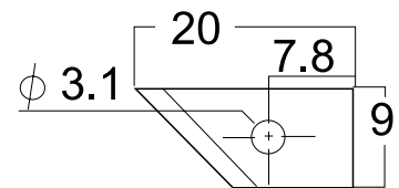
NT 圓形鋸刀刀片 NT Blade for C1500
